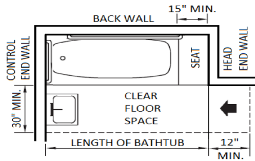
(d) PERMANENT SEAT IN TUB - SIDE APPROACH
