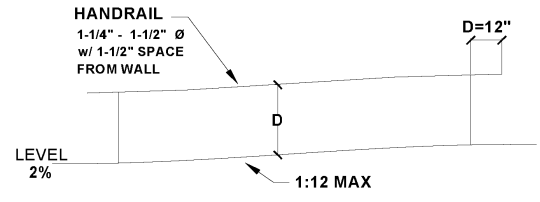
RAMP ELEV.
